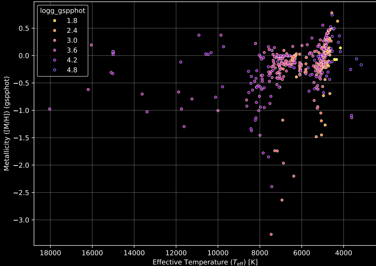
APOGEE DR17 Field: [120+04] Stellar Population Parameters (n= 431)
